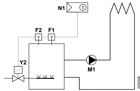
Atmosphärischer Gasbrenner
