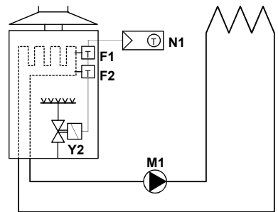
Warmwasser-Umlaufferhitzer (Heiztherme)
